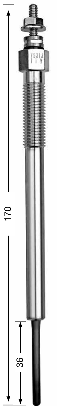
Y-531 J M 10 x 1.25 12 Hex 11 V DP 44
