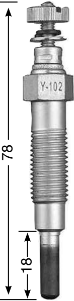
Y-102 M 10 x 1.25 12 Hex 10,5 V
