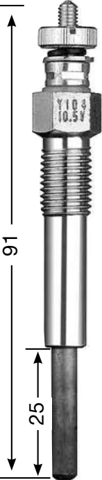
Y104 M 10 x 1.25 12 Hex 10,5 V
